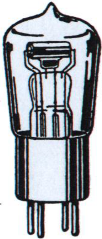
Fig. 47. Außenansicht der Loewe-Röhre.
